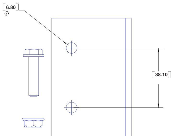
Кронштейн
